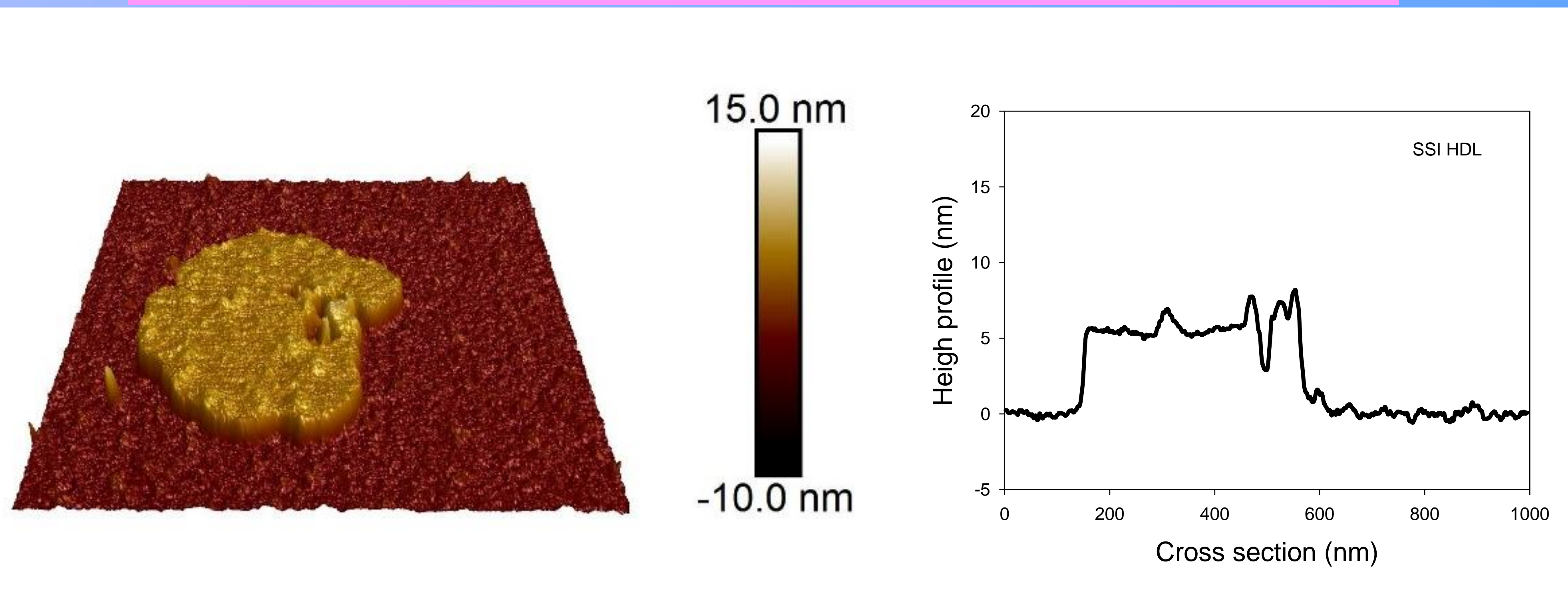
Caractérisation morphologique de SSI: exfoliation partielle des feuillets cationiques
