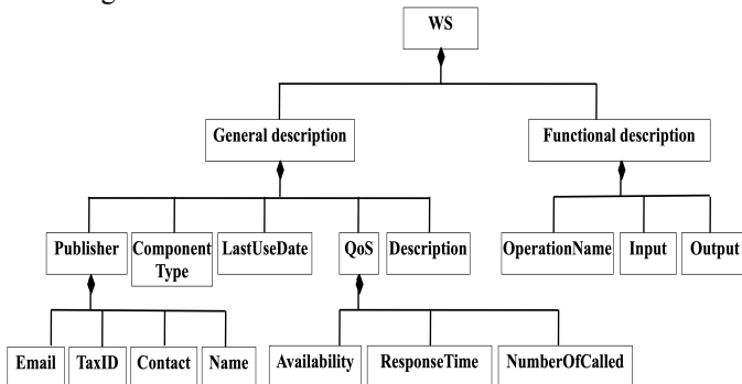
Fig. 10. Web service structure
