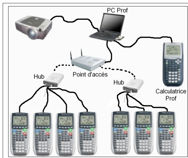
Figure 1 : le dispositif TI-Navigator
