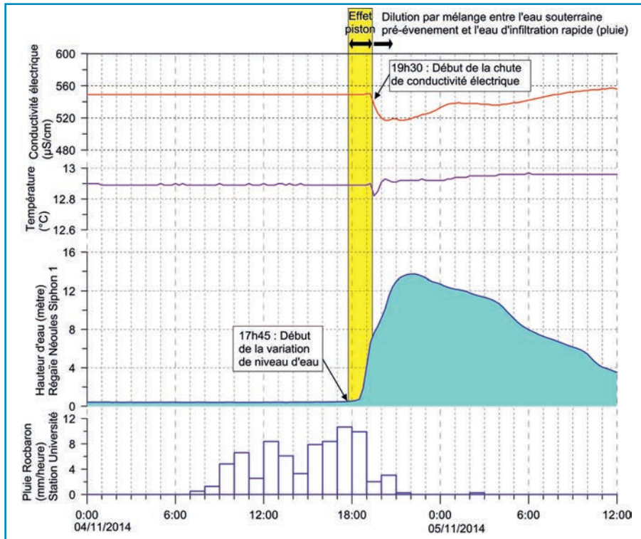
Figure 8: La crue du 4 et 5 novembre 2014 au Régaie de Néoules. Enregistrement des variations de hauteur d'eau, température et conductivité électrique de l'eau du siphon 1 au pas de temps de 15 minutes. Pluie horaire mesurée à Rocbaron. The flood of 4-5. November 2014 recorded in the sump 1 of the cave "Régaie de Néoules". Detailed CTD time-series (15 minutes' time-step) and rainfall per hour.
