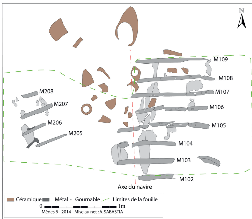
Figure 1. Plan de l'épave Médés 6. (M : membres).
