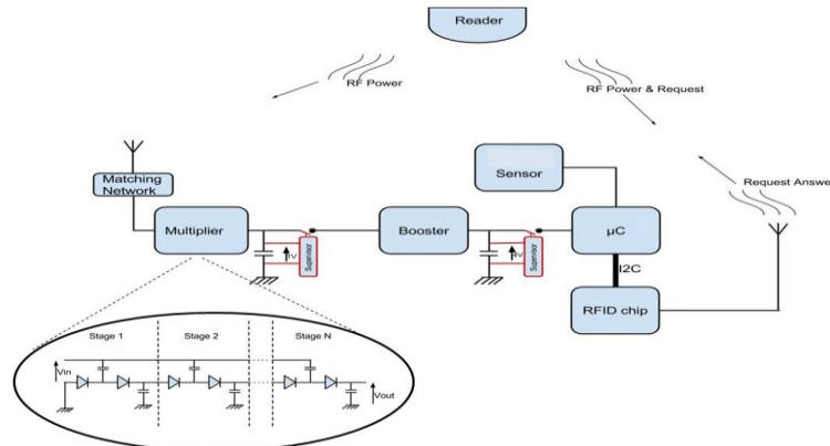
Figure 1, Architecture du système de récupération d'énergie
