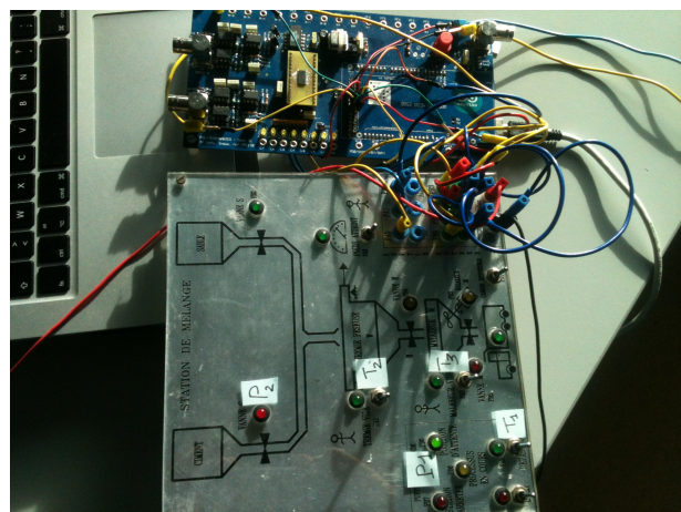
Fig. 4. Arduino card
