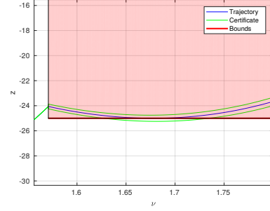
(d) Excursion of z-trajectory, RPAs of degree 7.
