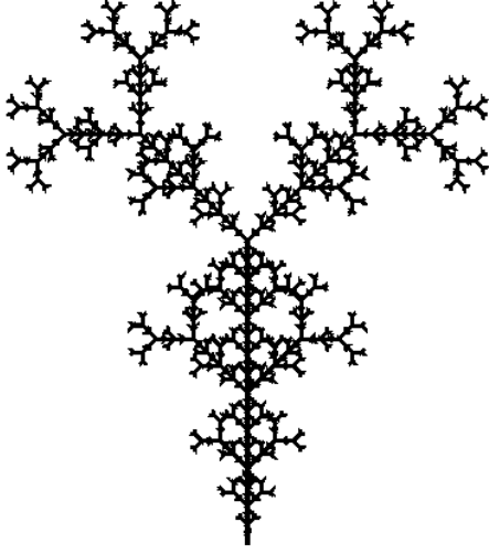
Figure 1: Exemple d'IFS composé de transformations affines dans le plan
