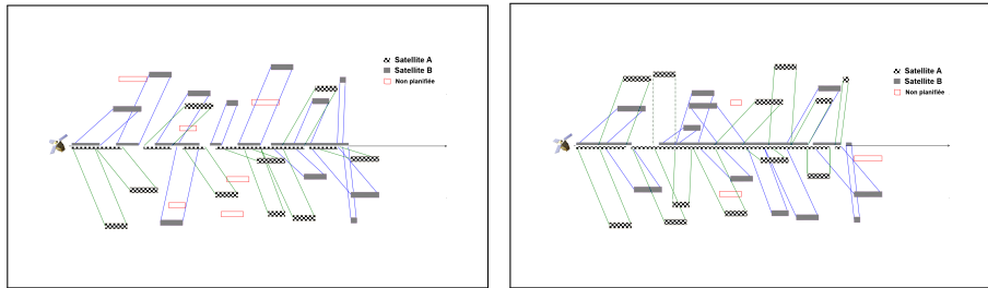
Figure 9. a et b. Comparaison de missions planifiées avec ChronoG (a) et ATLAS (b)
