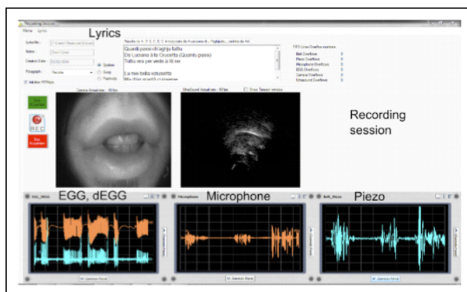
Figure 2. Capture d'écran du logiciel de session d'enregistrement (Chawah P, Al Kork et autres. 2014). En haut : affichage des paroles du chant enregistré. En-dessous : cinq images des capteurs synchrones, avec de gauche à droite et de haut en bas : image des lèvres captée par la caméra; contours de la langue tracés par l'échographie US; mouvements des plis vocaux captés par l'EGG; capture du son par le microphone (analyse spectrographique); capture des résonances nasales par l'Accéléromètre piézoélectrique.
