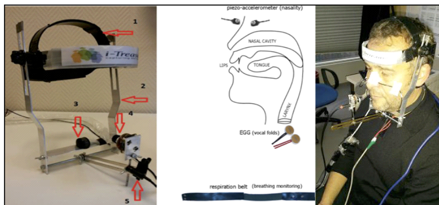
Figure 1. A gauche : l'hyper-casque à multi-capteurs (Al Kork et autres. 2014) comportant : 1) le bandeau réglable, 2) le support d'ajustement de hauteur, 3) la plate-forme de sonde échographique US réglable, 4) la caméra d'enregistrement des mouvements des lèvres avec le système d'ajustement de proximité et d'orientation, 5) le microphone. Au milieu : le schéma du placement des capteurs hors casque: Accéléromètre piézoélectrique (nez), l'EGG (plis vocaux) et la ceinture de respiration; A droite : photo du premier chanteur corse expérimentant l'hyper-casque dans notre laboratoire.
