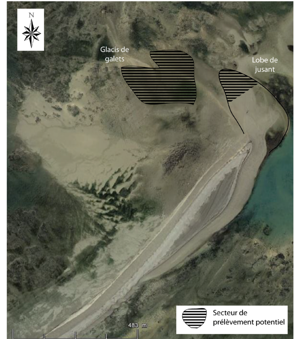
Figure 19 : Localisation des sites potentiels de prélèvement de galets pour le rechargement de la "taille de guêpe"
