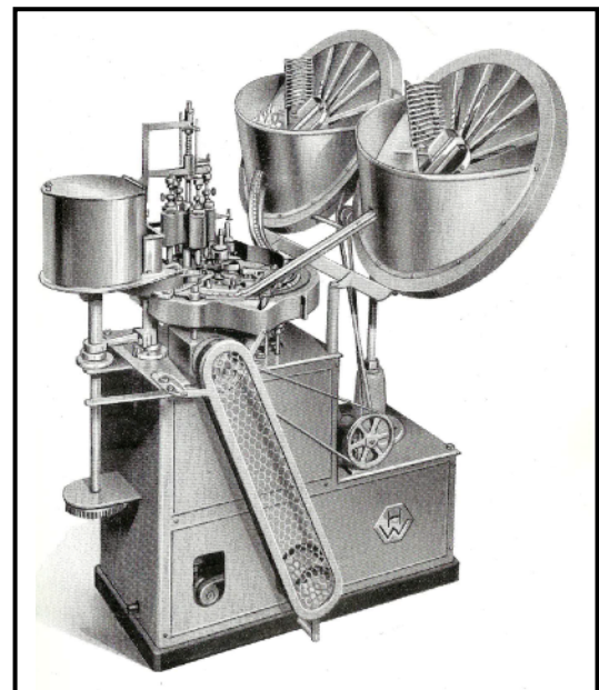
Modèle DS pour cachets emboîtés Laboratoires Midy (Paris)
