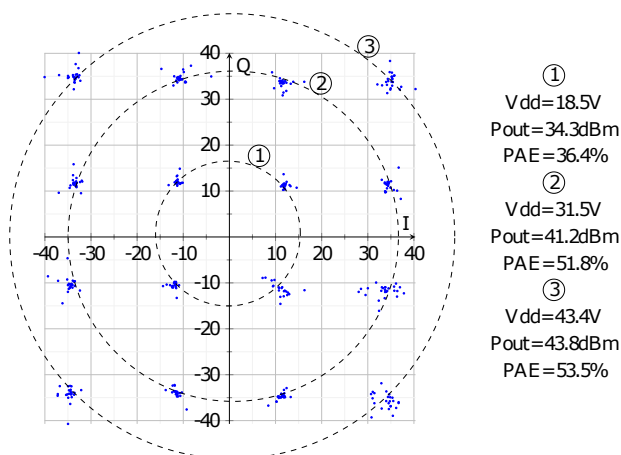
Figure 9. Constellation 16-QAM mesurée avec un débit de 40 Msymboles/sec pour une puissance d'OL de 19 dBm. Une correction d'amplitude et de phase appliquée en entrée permet d'obtenir un EVM de 3.2% avec un rendement global moyen de 38.1% [7].
