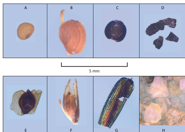
Fig. 4 - Exemples de macro-restes issus de la tourbière de La Narce du Béage : A - graine de Ranunculus – Ranunculus type Batrachium ; B - graine de Potamogeton sp. ; C - capsule de sporophyte de Sphagnum – Sphagnum sp. ; D - fragments de micro-charbon de bois, cf. Pin – Pinus ; E - graine de Betula pubescens – Betula pubescens ; F - semence de Poaceae , cf. Vulpin fauve – Alopecurus aequalis ; G - élytre de Coléoptère ; H - ensemble de particules minérales – quartz. Clichés A.-M. Dendievel.
