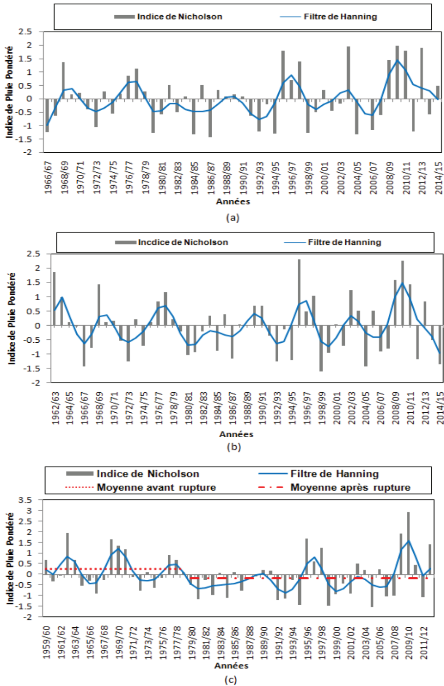
Figure 2 : Evolution interannuelle de la pluviométrie à Mechra Bel Ksiri (a), Azib Es Soltane (b) et M'jara (c) avec les indices centrés réduits des hauteurs de pluie et les totaux pluviométriques annuels pondérés.
