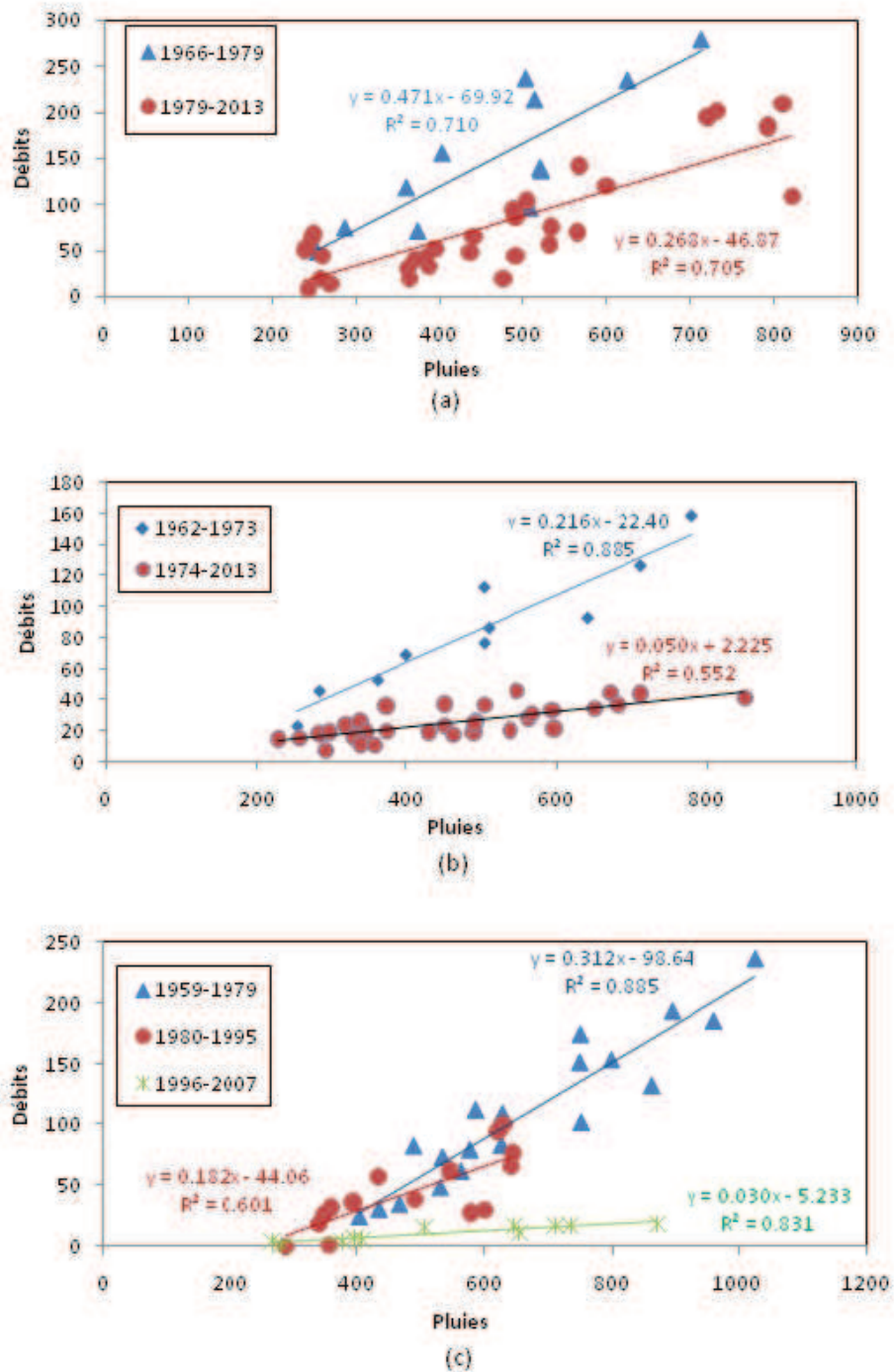
Figure 4 : Relations débits liquides-précipitations mesurés sur le Sebou à la station de Mechra Bel Ksiri (a), Azib Es Soltane (b) et M'jara (c).
