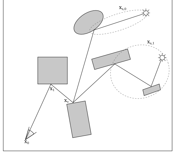
Figure 2: La séparation d'un chemin en trois parties. Ici, il y a une VPL géométrique, et deux VPLs virtuelles de chemin. On voit bien l'aggrégation des VPLs de chemin partageant le même point \mathbf{x}_v .
