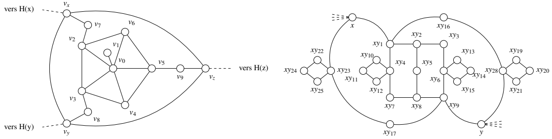
(a) Gadget H(v) pour un sommet v avec N(v) = \{x, y, z\} dans G (b) Gadget I(x, y) , planaire, biparti et de degré maximum 4.
