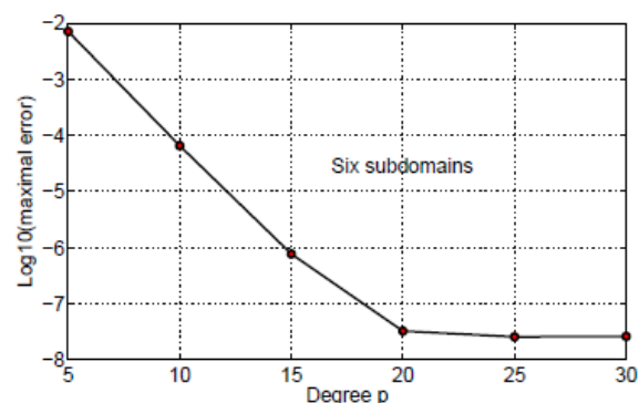
Figure 1 – Exemple de convergence exponentielle pour une résolution en six morceaux
