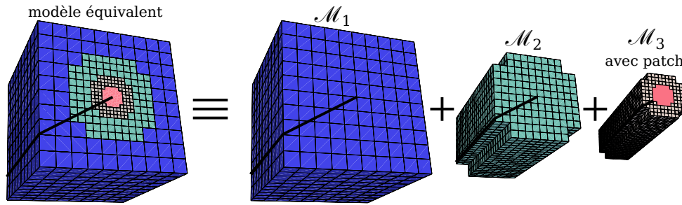
FIGURE 3 – Représentation de la discrétisation multigrilles localisées avec le patch en rouge.
