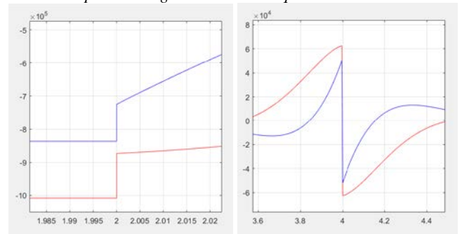
Fig. 23: Zooms sur l'interface air/tôles de la Fig. 22, puis sur le premier inter-tôles, montrant les fausses discontinuités du champ introduites par l'homogénéisation classique :
