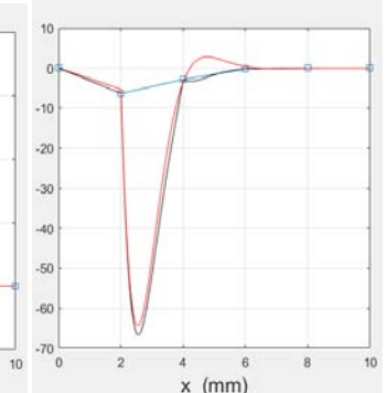
Fig. 20: Solution homogénéisée
