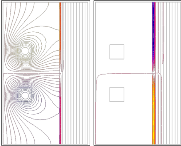
Fig. 39 : 10Hz, mur= 10000
