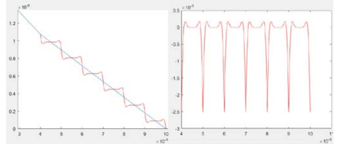
Fig. 32: Même cas, tôles en court-circuit
