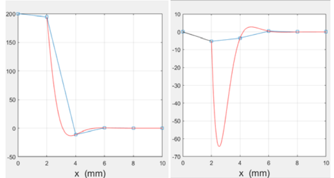
Fig. 18: 1 kHz, solution homogénéisée suivant [1] :
