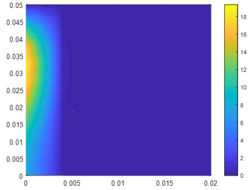
Fig. 43 : Erreur en % avec l'homogénéisation classique (calculée par rapport au maximum du module du pot. vecteur).
