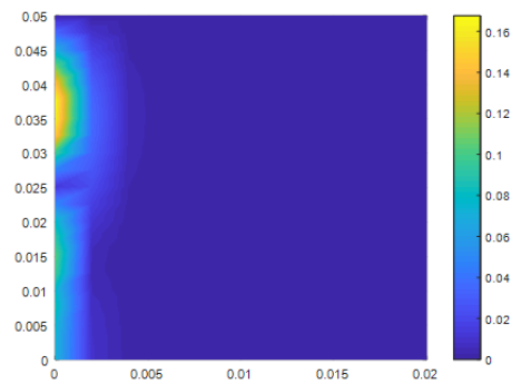
Fig. 41 : Erreur relative en % (de max) / référence
