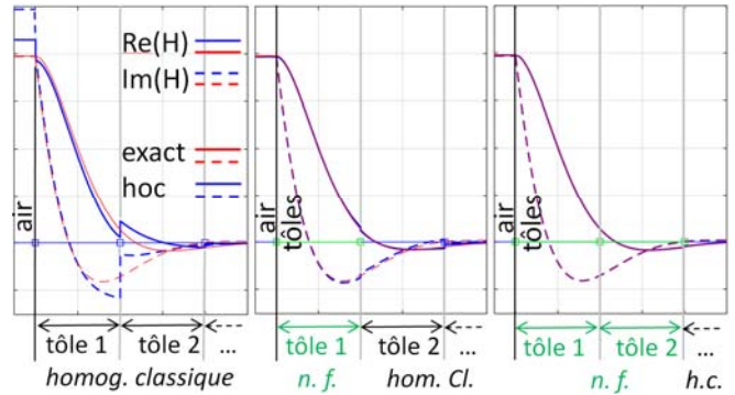
Fig. 3 : Mélange de formulation : 2 tôles en « nouvelle formulation » suffisent pour converger vers la solution exacte (toutes les tôles en « nouvelle formulation »). Système à 40 tôles, maillage élargi à partir de la tôle 7.
