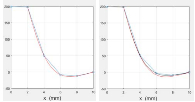
Fig. 15: 100 Hz, \mu_r=100
