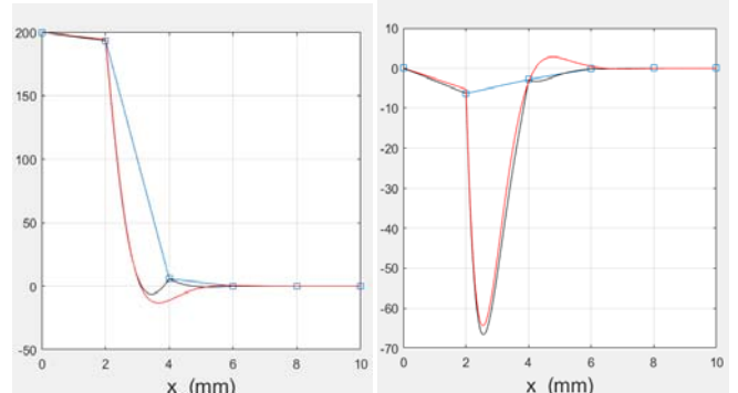
Fig. 19: 10 kHz
