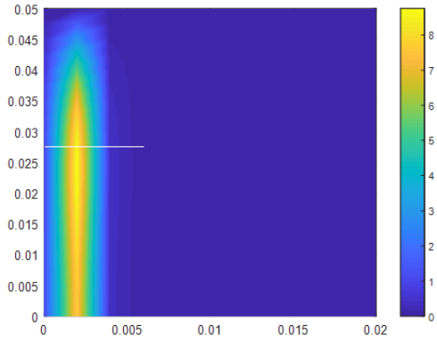
Fig. 44 : 100Hz, mur=1000.
