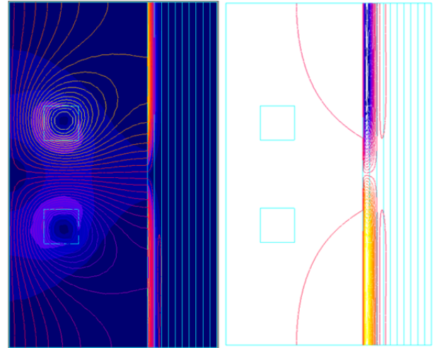
Fig. 45 : 25Hz, mur=1000, hom. Classique : max 6,5%
