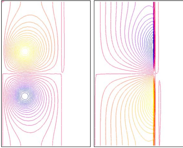
Fig. 42 : 100000Hz, mur=1
