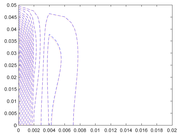
Fig. 37 : Parties réelles (en haut) et imaginaires (en bas) du pot. vecteur tracées sur la moitié supérieure des tôles : sur chacune des deux vues, comparaison entre Flux2D (valeurs de référence via maillage très fin, pointillés rouges) et la nouvelle formulation (tirets bleus), en ne retenant (pour Flux) que les valeurs aux inter-tôles. Mêmes échelles de valeurs pour les 2 méthodes.
