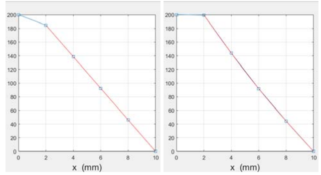
Fig. 15: 100 Hz, \mu_r=100
