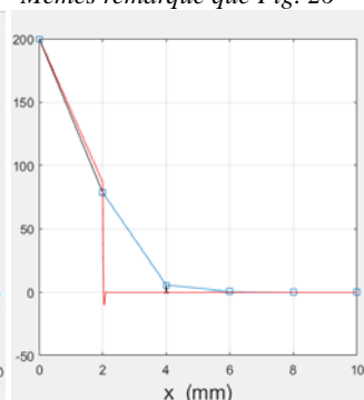
Fig. 28: Solution hom. [1]: Mêmes remarque que Fig. 26
