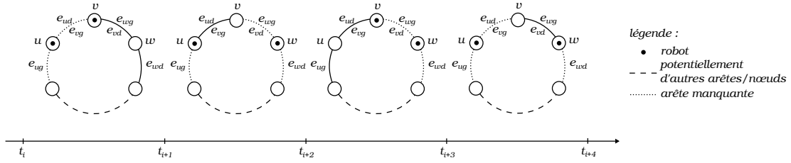
FIGURE 2: Construction de G_i , G_{i+1} , G_{i+2} , et G_{i+3} (preuve d'impossibilité avec deux robots).
