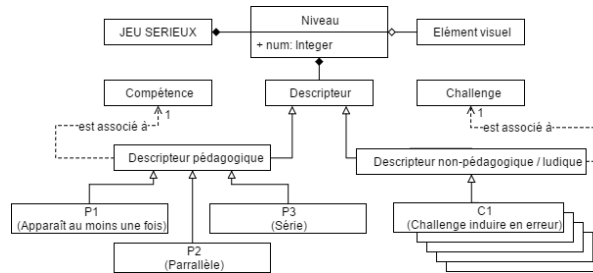
Figure 3. Le modèle UML simplifié d'un niveau vu selon l'angle de nos descripteurs
