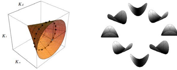
FIGURE 1 – a) Le cône \det K = 0 dans le cas isotrope ( \eta = 0 ) ; b) Configurations stables cylindriques.
