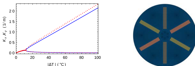
FIGURE 3 – a) Bifurcation du champ de courbures (trait plein : Abaqus ; trait pointillé : Von Kármán). b) Disposition des actionneurs sur le disque et maillage éléments finis.
