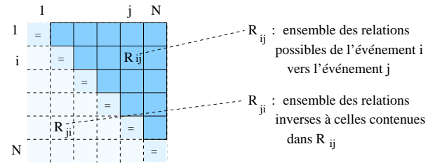
FIG. 9 – Les relations entre N événements sont stockées dans la matrice Triangulaire (N-1) \times (N-1) .
