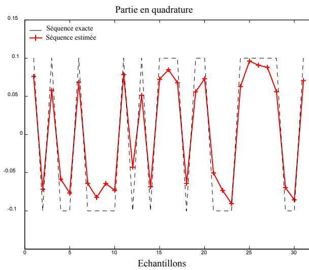
FIG. 11: Séquences en quadrature
