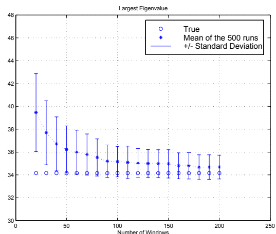
Fig. 11 : Monte Carlo simulations
