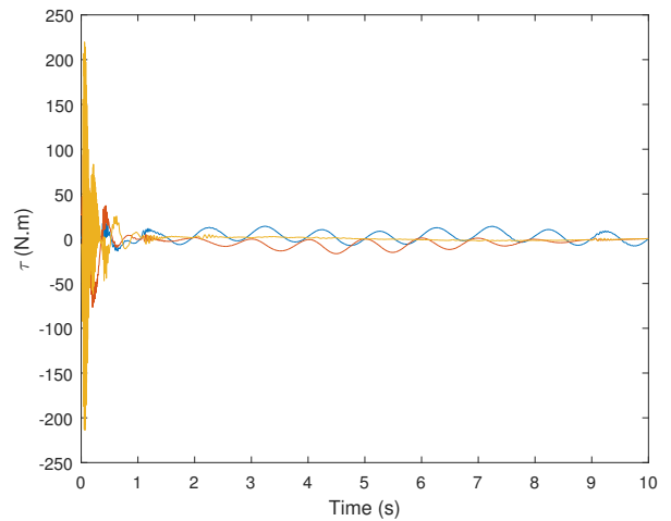
Fig. 3: Input torques \tau
