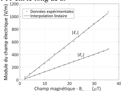
Figure 1: Module du champ E radial |E_r| et longitudinal |E_z| en fonction de l'amplitude du champ magnétique RF.
