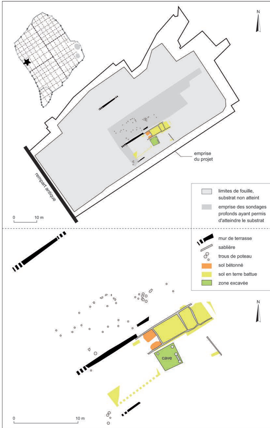
Fig. 7 – Nouvel hôpital (2001) : plan de l'état augustéen (DAO : Y. Labaune, ArTeHis, d'après Ph. Bet).
