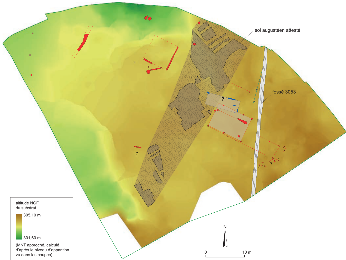
Fig. 6 – Faubourg d'Arroux (2010) : plan de l'état augustéen (DAO : St. Alix, Inrap).
