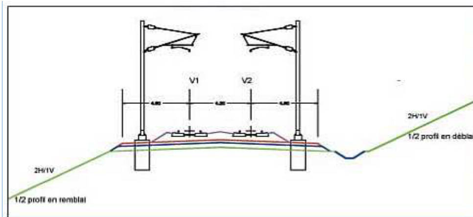
Illustration 3: Profil en travers type d'une structure ferroviaire (d'après « Liaison ferroviaire Lyon-Turin » document public RFF)
