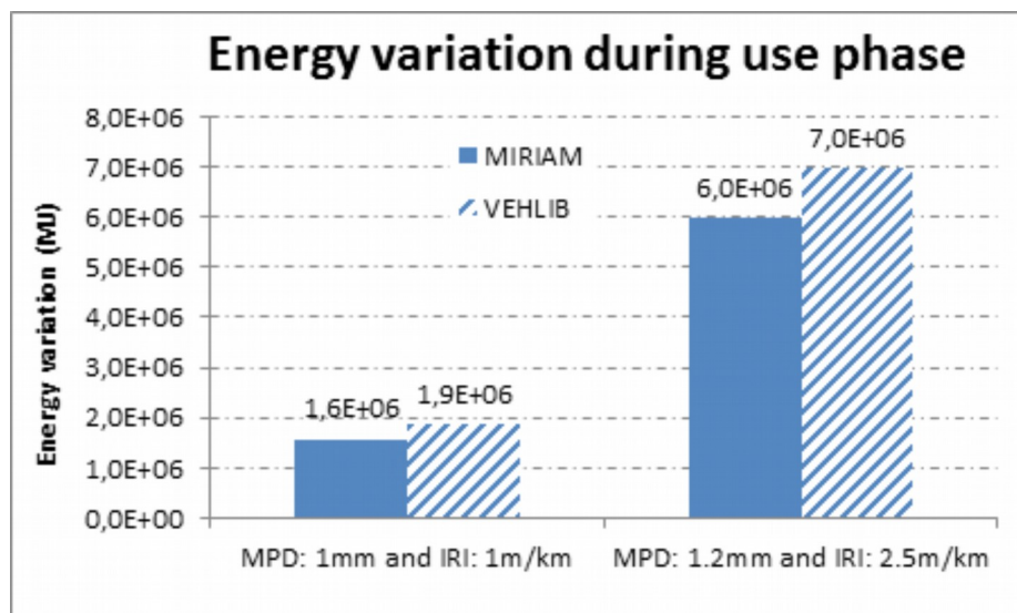
Illustration 14: Consommation d'énergie pendant la phase d'usage en fonction de la macrotexture et de l'uni (Cerezo et al., 2016)
