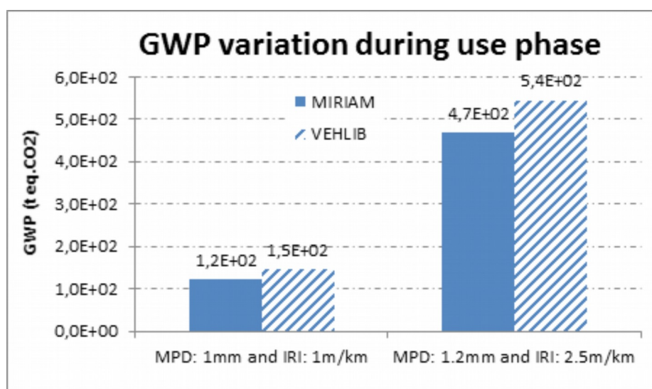
Illustration 15: Émissions de GeS pendant la phase d'usage en fonction de la macrotexture et de l'uni (Cerezo et al., 2016)
