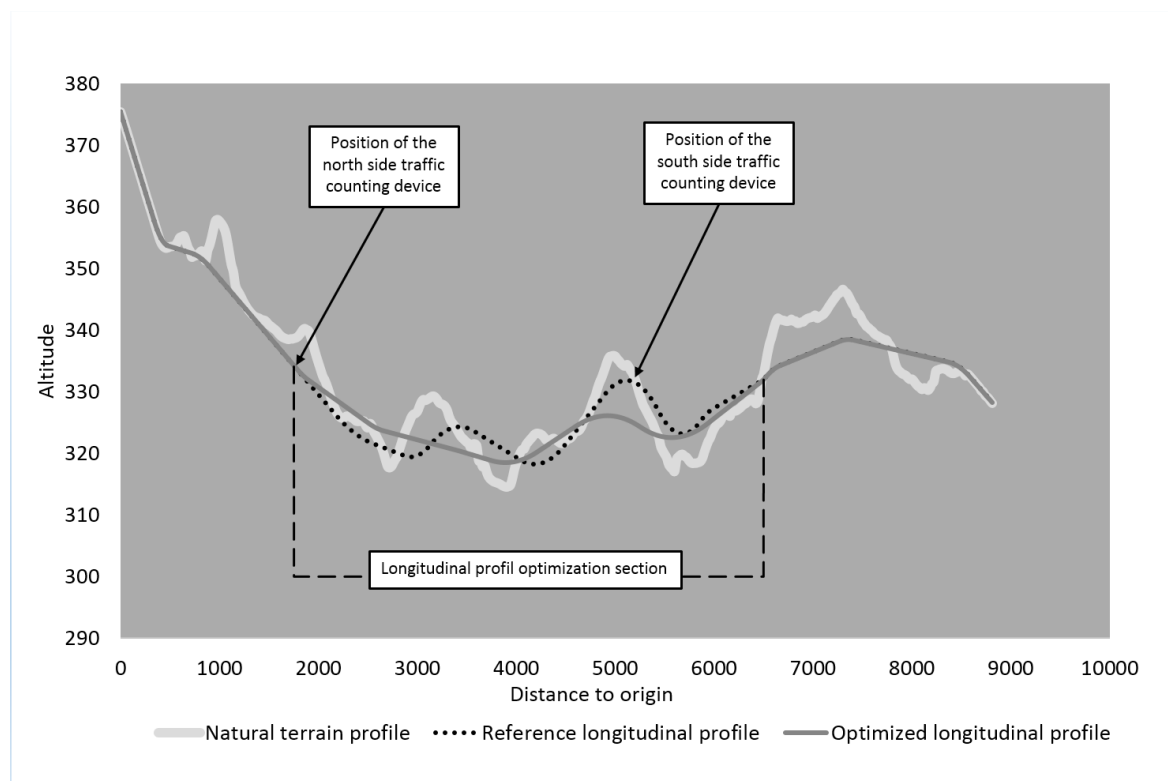
Illustration 12: Terrain naturel, profil de la route, profil optimisé
