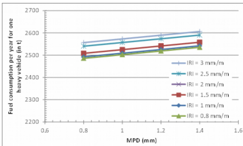
Illustration 13: Consommation annuelle d'un poids lourd en fonction de l'uni (IRI) et de la macrotexture (MPD) (Cerezo et al., 2016)
