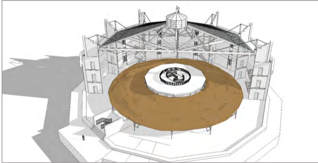
Fig 7 Coupe révélant le faux-terrain - ill.Lescop – 2016
