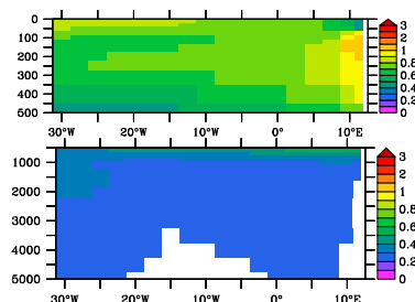
PISCES 1, CoFeMUG
