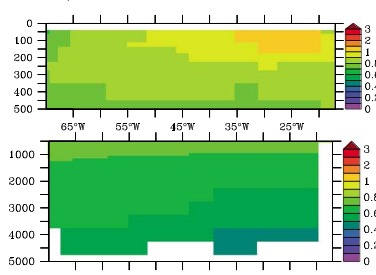
MITecco, GA-03
