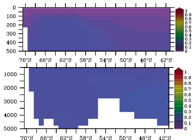
GENIE, GIPY-5
