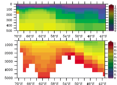
PISCES 2, GIPY-5
