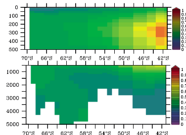
PISCES 1, GIPY-5
