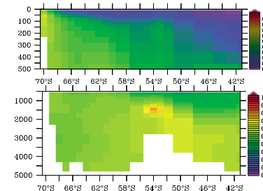
TOPAZ, GIPY-5
