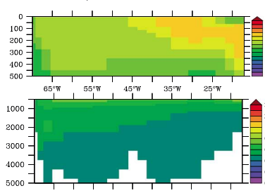
MITgsm, GA-03
