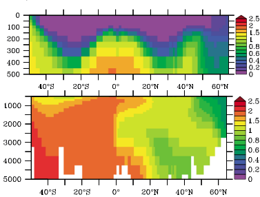
GENIE, GA-02
