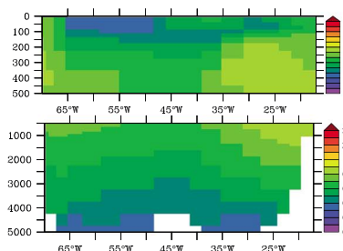
MEDUSA 1, GA-03
