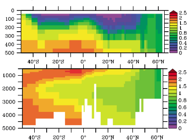
MITecco, GA-02
