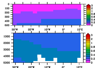
GENIE, CoFeMUG
