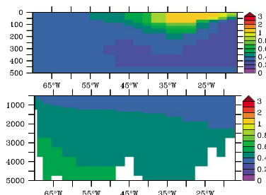
GENIE, GA-03
