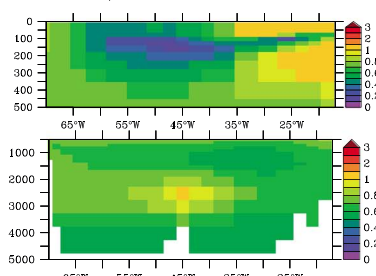
PISCES 2, GA-03
