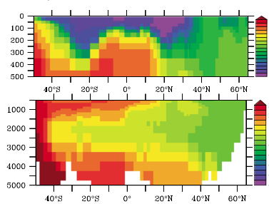
MEDUSA 1, GA-02
