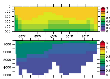
PISCES 1, GA-03
