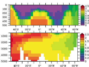
PISCES 2, GA-02
