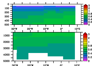
MITecco, CoFeMUG
