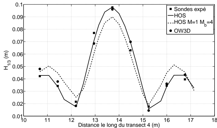
FIGURE 5 – Hauteur crête à creux le long du Transect 4 - houle régulière - cas M1 avec H_0 = 0.0465\text{m} et T_0 = 1.3\text{s} - Comparaisons HOS/OW3D.
