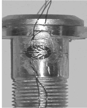
Fig. 14 Instrumented bolt.
