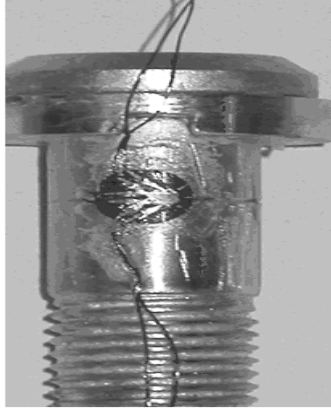
Fig. 14 Instrumented bolt.
