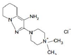
R0069603A: MW 285.82
