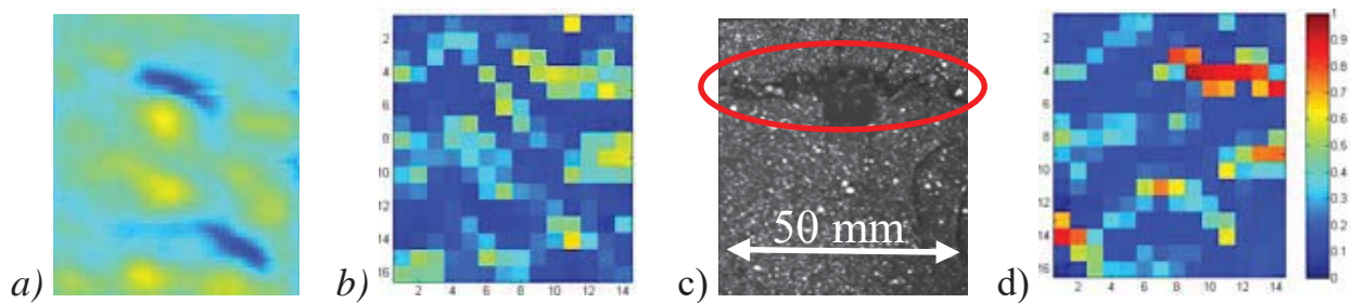
Figure 4. a) Contrastes d'amplitudes ultrasonores (C-scan en transmission) avant l'essai b) contrastes de modules identifiés à partir des champs de déplacements en début d'essai c) faciès de rupture d) carte identifiée à partir de l'avant dernière image saisie avant rupture
