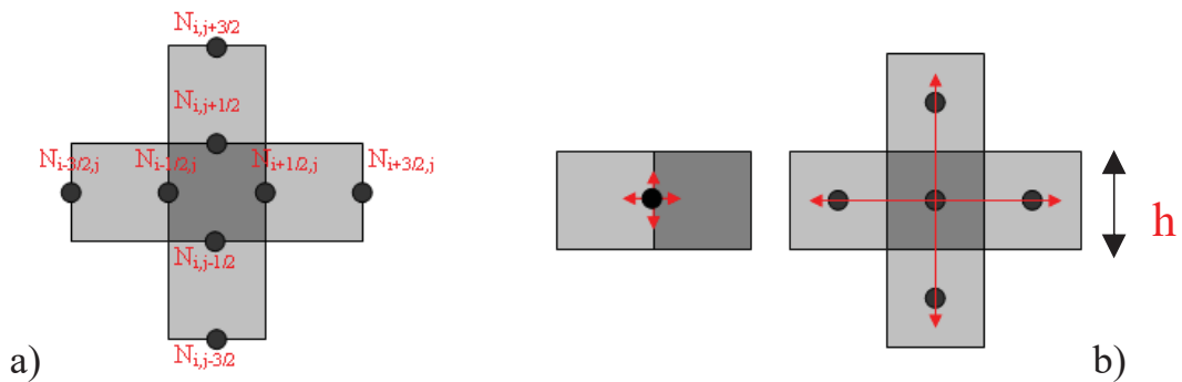
Figure 1. a) Numérotation des nœuds autour d'un élément K_{i,j} b) Ecriture de l'équilibre aux frontières et au centre de l'élément.
