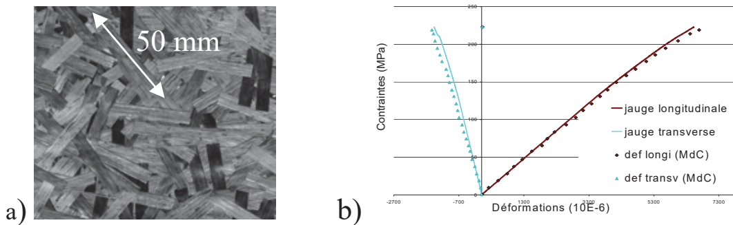
Figure 3. a) Répartition aléatoire des bandelettes de carbone dans un pli (HexMC ® ) b) Comparaison de déformations mesurées par jauges et par mesure de champs au cours d'un essai de traction (sens longitudinal et transversal)
