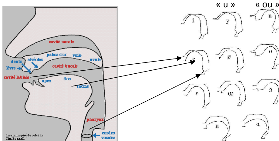
Figure 1 : A gauche, coupe schématique du conduit vocal A droite : formes du conduit vocal pour l'articulation des voyelles du français.
