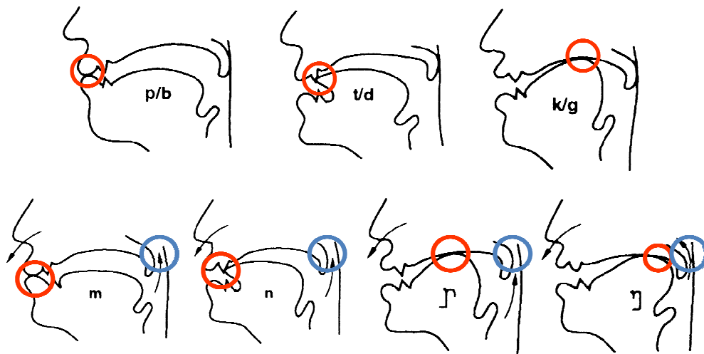
Figure 2 : Formes du conduit vocal pour l'articulation de certaines consonnes du français. En haut les consonnes occlusives (orales), en bas les consonnes nasales.
