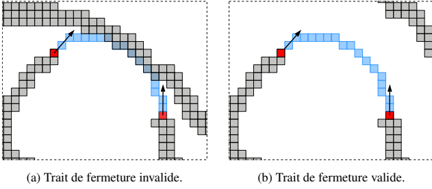
FIG. 7: Configurations de fermeture par courbe spline sur une partie d'image I_f (en gris). En (a) la courbe spline \mathcal{S} (en bleu) issue des deux points d'intérêt (en rouge) est telle que \tau(\mathcal{S}, I_f) = 4 , elle n'est donc pas ajoutée. En (b) on a \tau(\mathcal{S}, I_f) = 2 , la courbe peut donc être dessinée.
