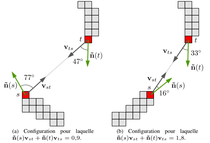
FIG. 6: Illustration de second terme du facteur de qualité \omega(s, t) . La configuration (b) est jugée plus favorable à la fermeture par une courbe spline que la configuration (a).
