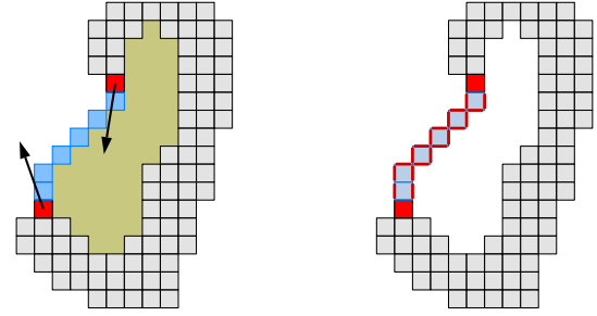
(a) Courbe spline créant une région de petite taille, en marron (48 pixels). (b) Lignels à partir desquel un suivi de contour est effectué.
