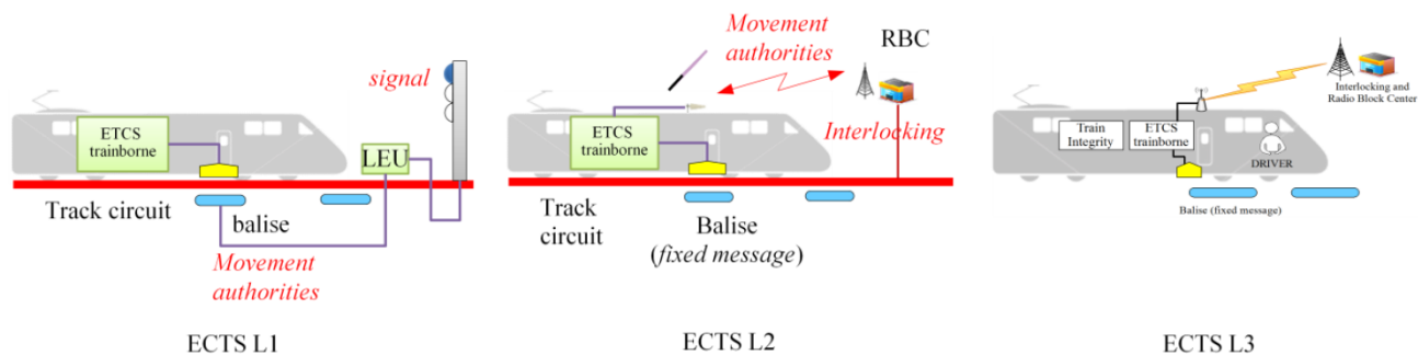
Fig. 2. ETCS Levels [86].
