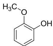
Guaiacol
