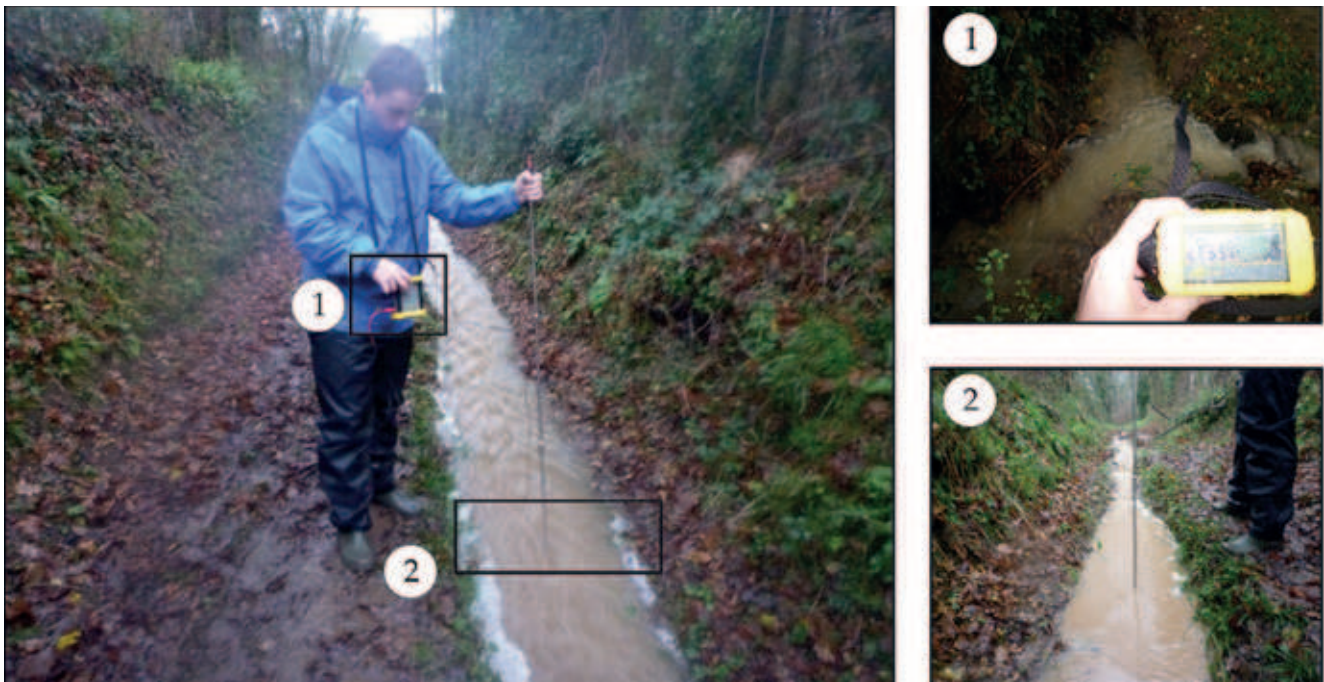
▲ Mesure des débits au moulinet.
