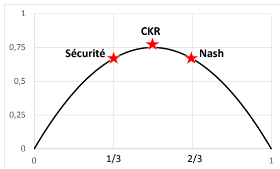
Les espérances de gain des différents équilibres (en fonction de p)
