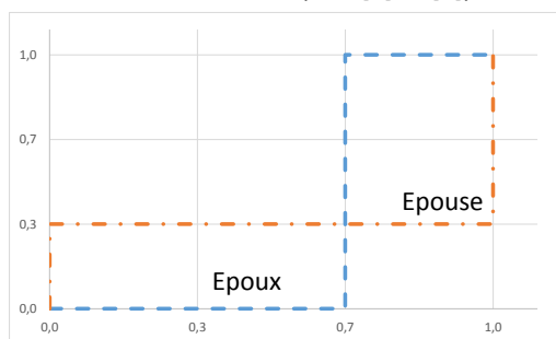
Equilibre de Nash (en fonction de la probabilité de foot)
