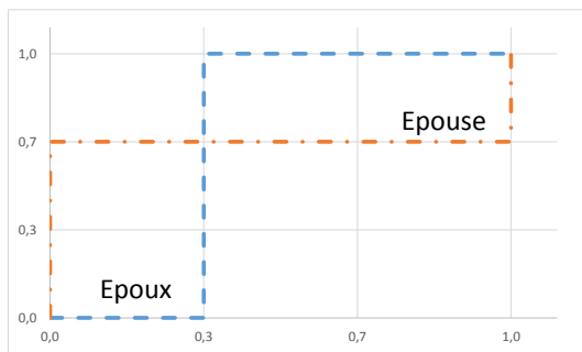
Equilibre sans CKR (en fonction de la probabilité de foot)
