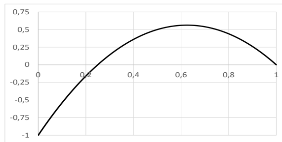
Espérance de gain sous CKR – variante (en fonction de p)
