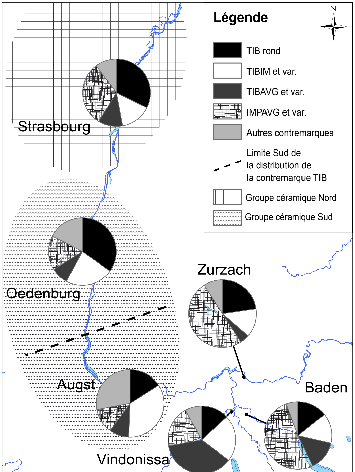
Fig. 7 [p. 155] : Répartition des différents types de contremarques tибériennes sur le Rhin supérieur, avec indication des groupes céramiques définis par M. Zehner (2002). (DAO : S. Martin.)
