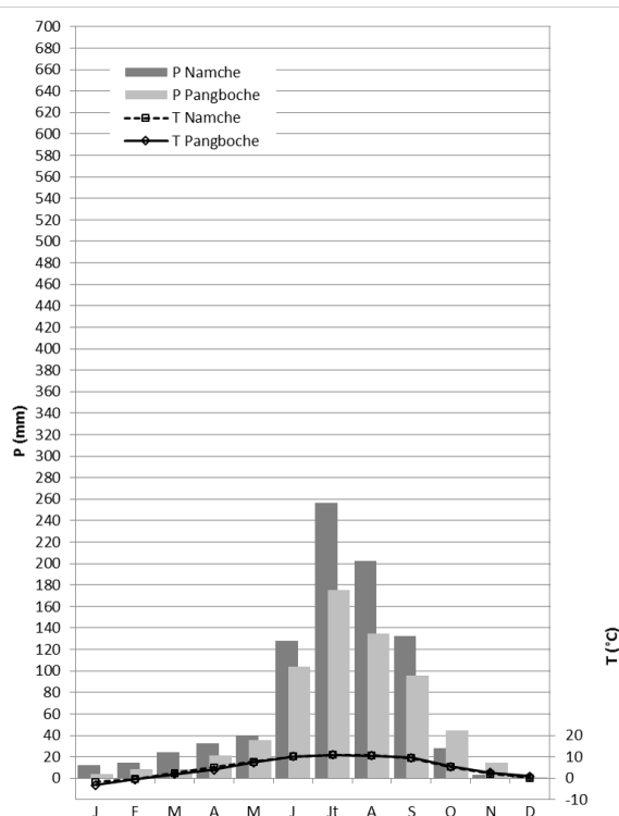
Figure 4. Diagrammes ombrothermiques. Haute Montagne
