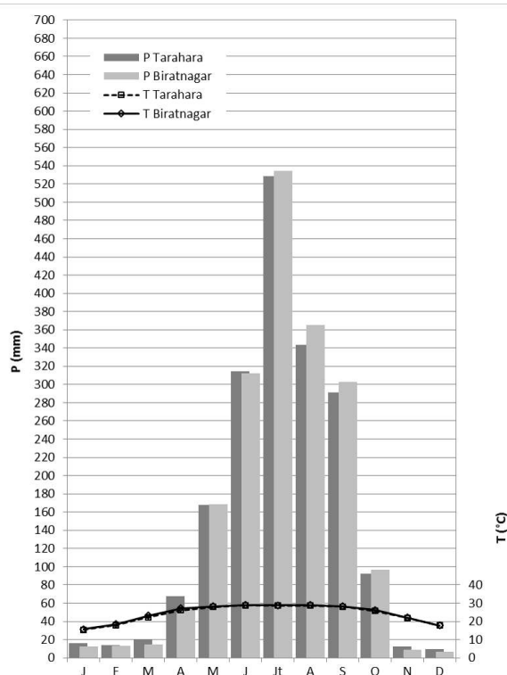
Figure 10. Diagrammes ombrothermiques. Plaine du Térai
