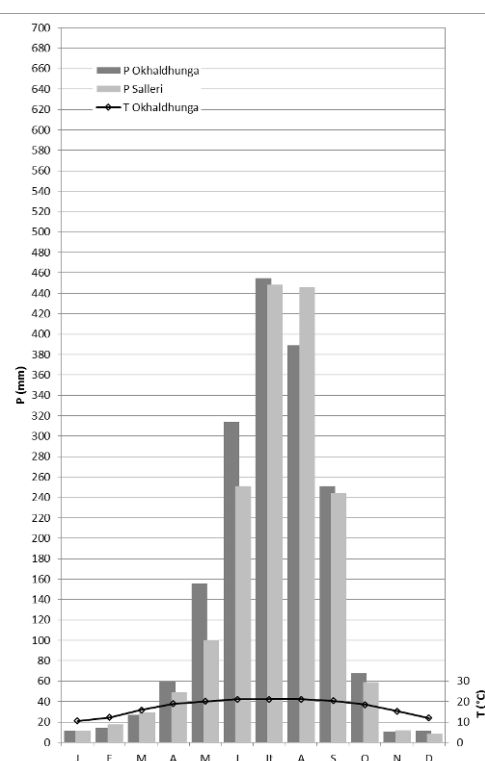
Figure 8. Diagrammes ombrothermiques. Basse Montagne
