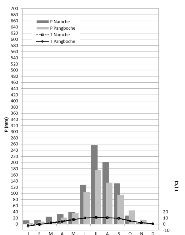
Figure 4. Diagrammes ombrothermiques. Haute Montagne
