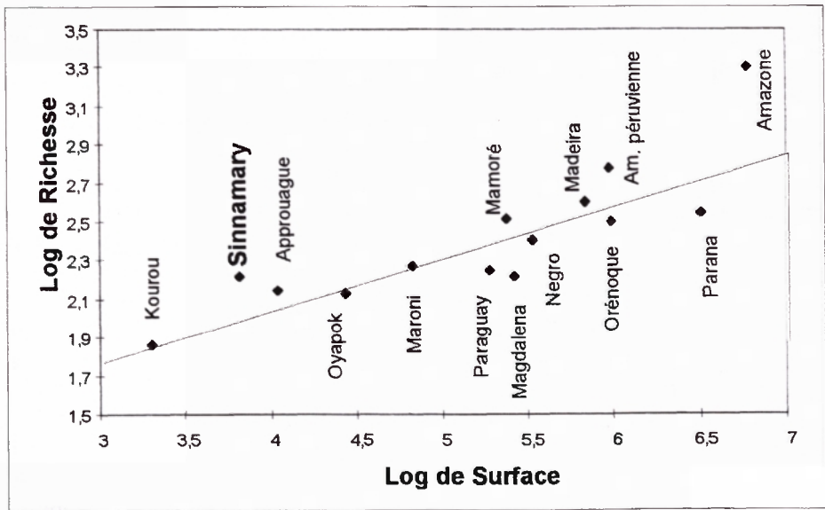
Fig. 2. – Relation entre la taille des bassins et la richesse spécifique des poissons pour quelques fleuves et rivière d'Amérique du Sud. Modifié de Lauzanne et al. (1993).
