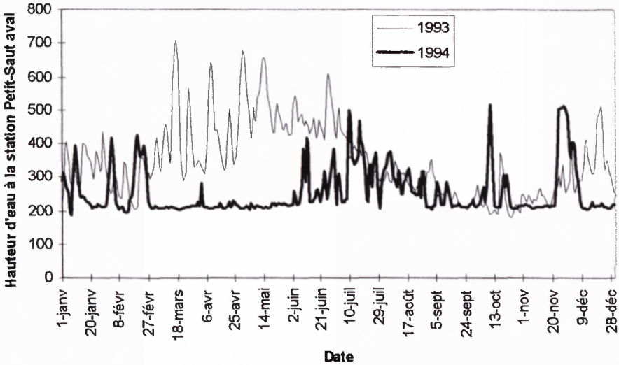
Fig. 6. – Variations des hauteurs d'eau journalières à la station limnimétrique de Petit-Saut Aval en 1993 et 1994.
