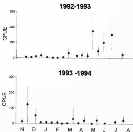
Fig. 5. – Variations des captures par effort de juvéniles dans les nasses lumineuses pendant les saisons 1992/93 et 1993/94 dans la crique Vénus (affluent rive droite de Sinnamary à l'aval du barrage de Petit-Saut). D'après Ponton (1995).
