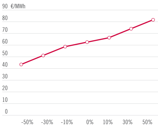
Figure 4. Évolution du coût de production en fonction des variations du coût d'investissement par kW (€/MWh)
