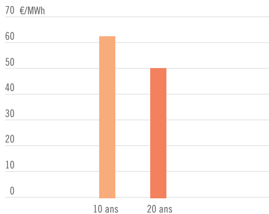
Figure 5. Évolution du coût de production en fonction de la durée de vie additionnelle
